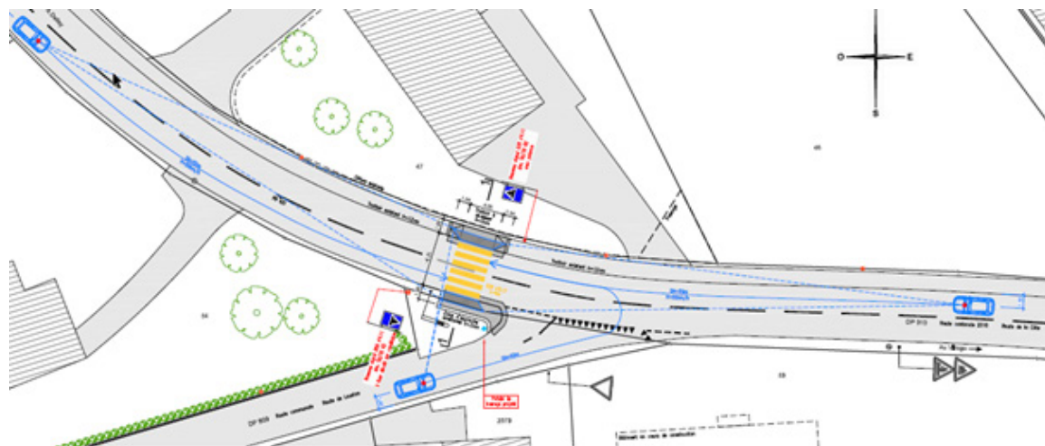
Route de la Côte –Projet d'aménagement d'un passage pour piétons
