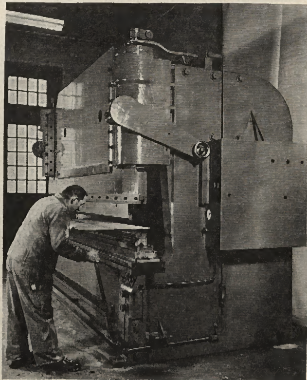
Travail à la presse à profiler la tôle.
