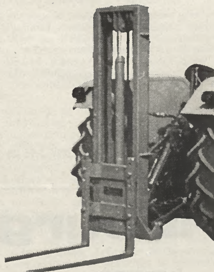
Elévateur à fourche à monter sur le relevage du tracteur
