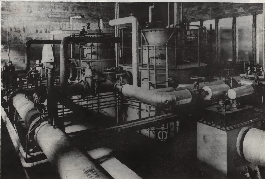
Réacteur et surchauffeur de vapeur de l'usine à gaz par craquage de l'essence légère (1968): deux lignes de production ayant chacune une puissance de 3500 kW.
