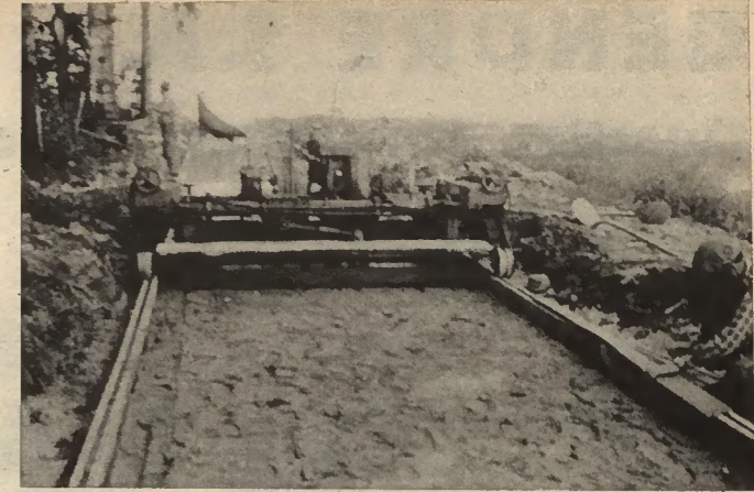
La construction de chemins en béton, solution économique. La finisseuse achève la mise en place du matériau.
