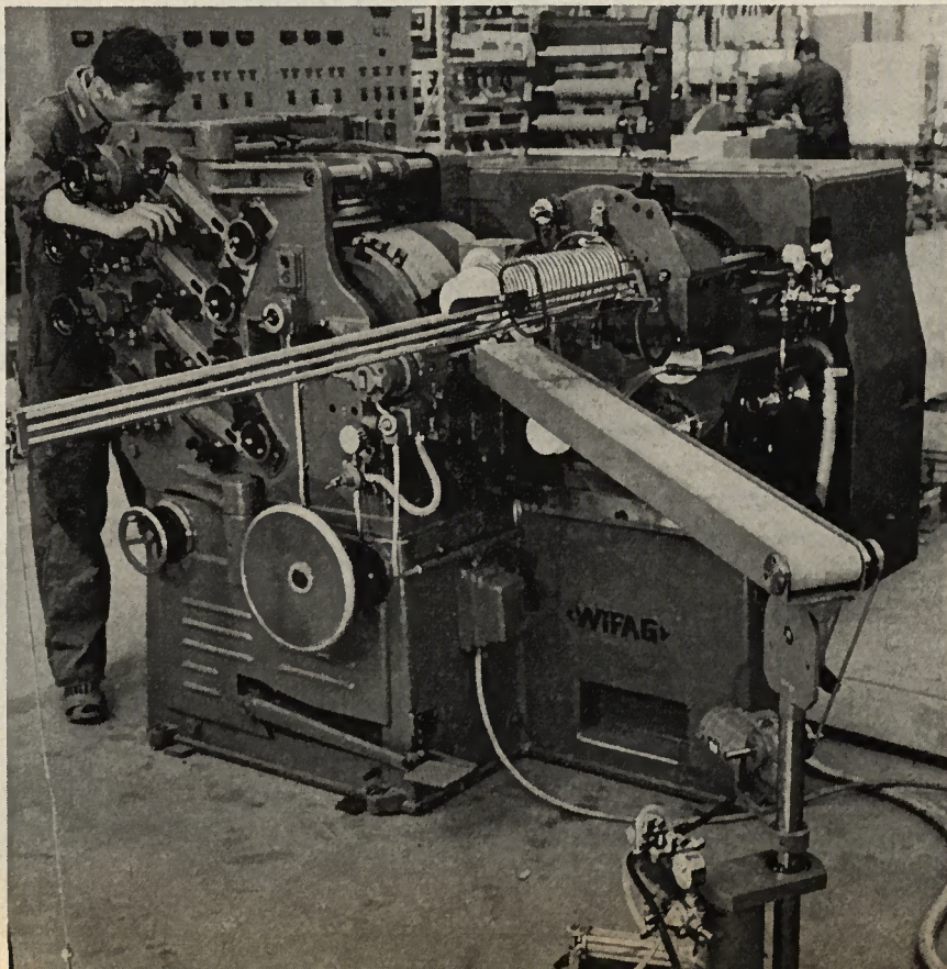
Montage d'une machine à imprimer les gobclets, munie d'un chargeur automatique.
