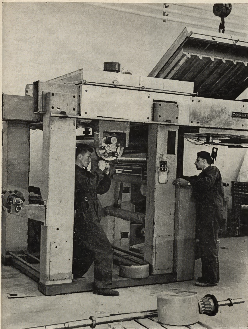
Chaque machine sortant des usines est montée, essayée et contrôlée. Deux monteurs occupés au montage d'une machine pour l'enduction et le contre-collage.
