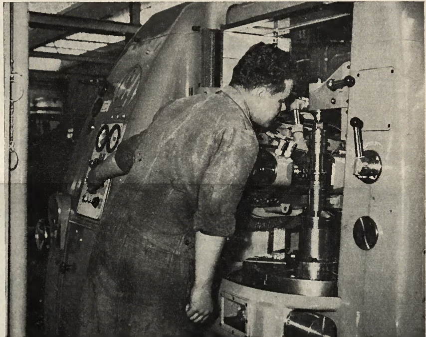
Fraisage par génération d'un pignon à chaîne sur une machine moderne.
