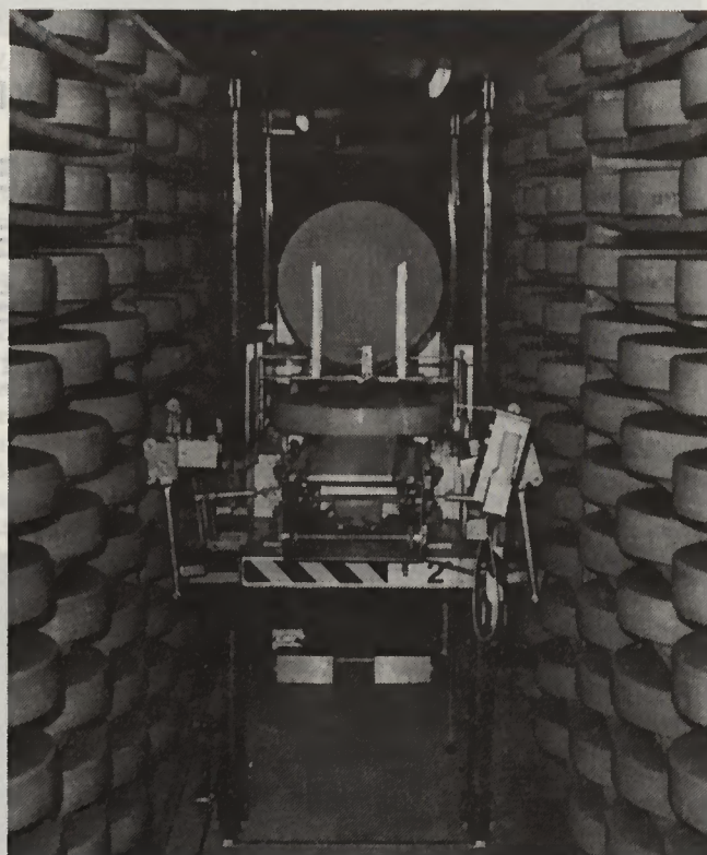
Le robot qui, jour et nuit, soigne les fromages.
