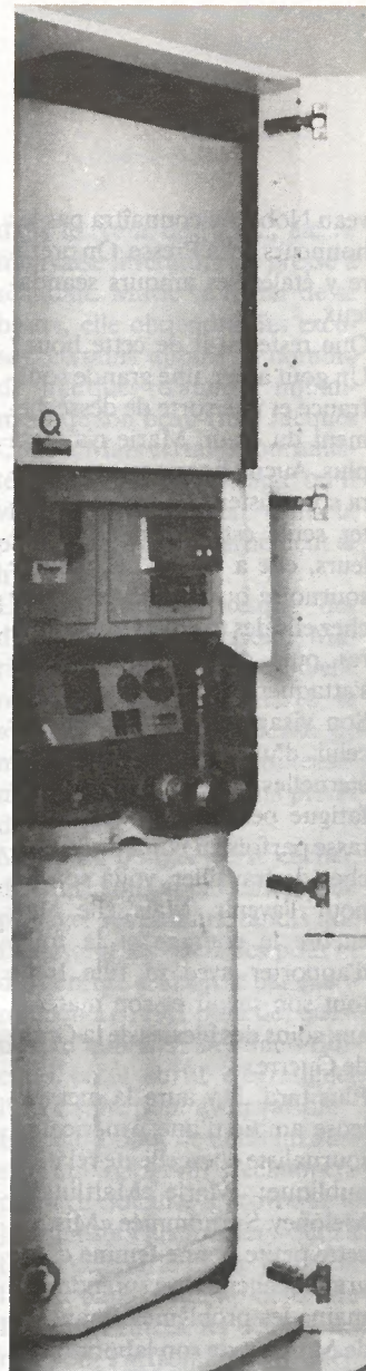
Chaudière à ventouse avec brûleur atmosphérique de 12 kW Low-NO x raccordée à une cheminée spéciale pour prise d'air frais et évacuation des produits de combustion (chauffage par appartement à la rue de Romont à Fribourg).
