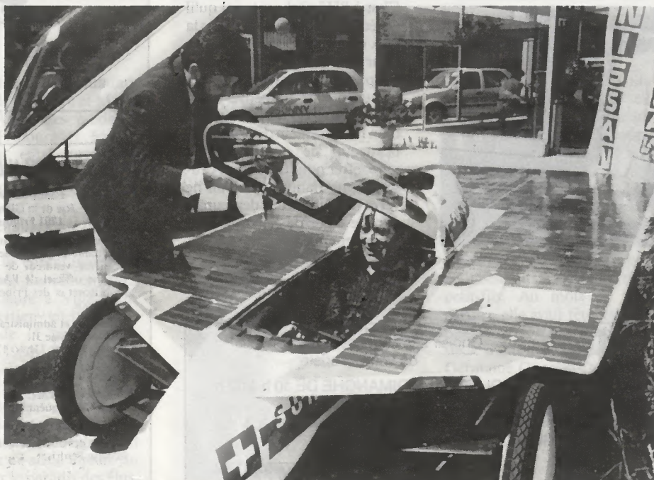
Un véhicule solaire pour individualiste forcené!
